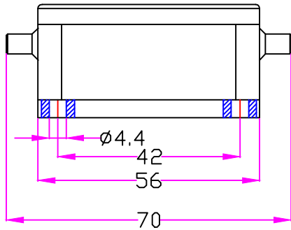
面板开孔图
