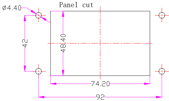
面板开孔图
